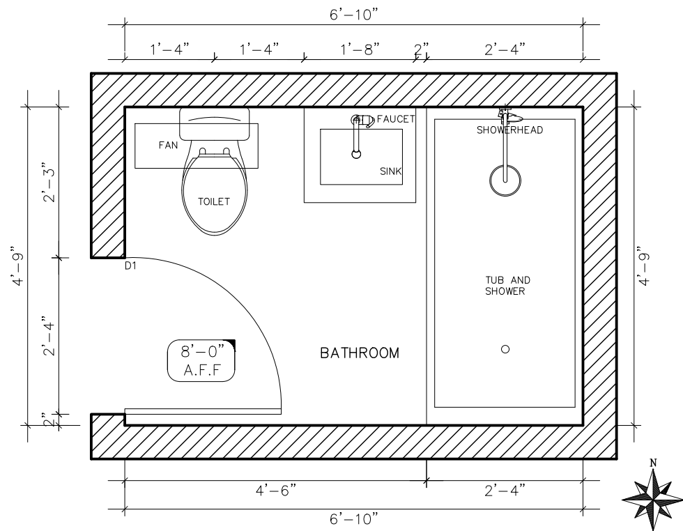
1 EXISTING FLOORPLAN 101 SCALE: 1/2" = 1'-0"
